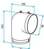
Codo 90° Ø 80 mm
