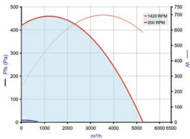
EasyVEC-Standard-4000
