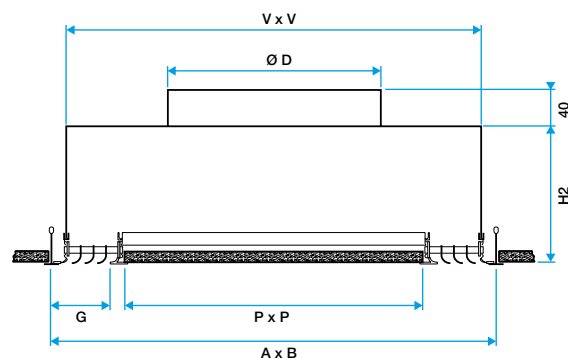
Diffuseur ALD 610K avec plénum piquage dessus
