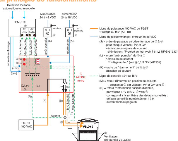
Esquema de principio de un ventilador de 1 velocidad desenfumage.
