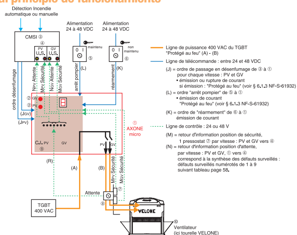
Diagrama esquemático de una instalación con una caja de 2 velocidades de desenfumaje.
