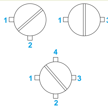
Schéma d'encembrement Collecteur Raccord d'Etage multilogement
