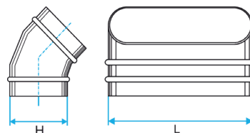
Esquema dimensiones Codo Vertical Oblongo 45°
