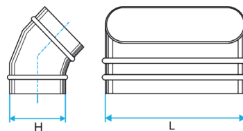
Esquema dimensiones Codo Vertical Oblongo 45°
