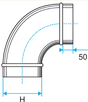
Esquema dimensiones Codo Vertical Oblongo 90°
