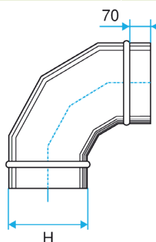
Esquema dimensiones Codo Vertical Oblongo 90°
