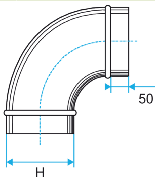
Esquema dimensiones Codo Vertical Oblongo 90°
