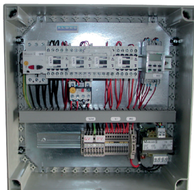
Coffret de desenfumage habitat collectif
