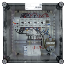
Coffret de désenfumage parking habitat collectif
