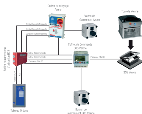
Esquema de principio cajetín de rearme AXONE y SOS VELONE
