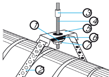
Esquema de instalación de la cinta perforada
