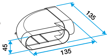
Coude horizontal 90°
