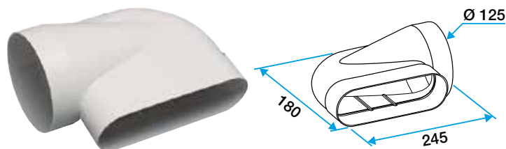
Codo 90° horizontal para conducto
