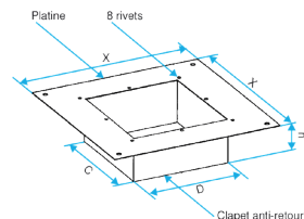
Compuerta antirretorno VELONE
