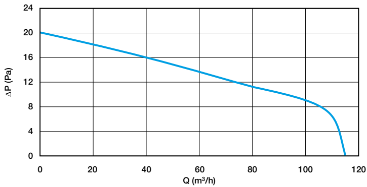
Curva aerológica DECO 125
