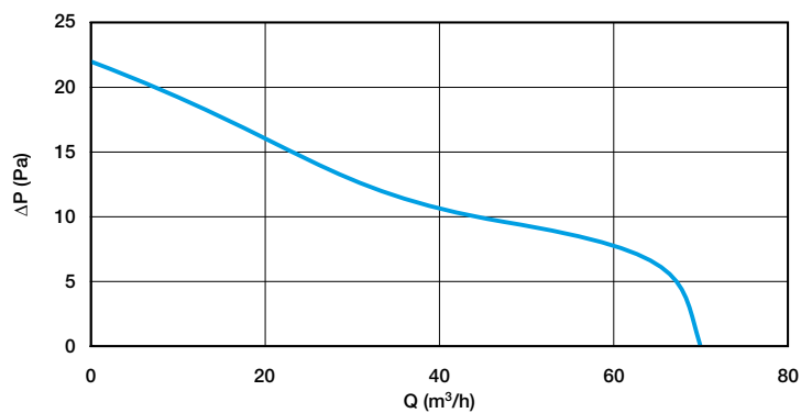
Curva aerológica DECO 100
