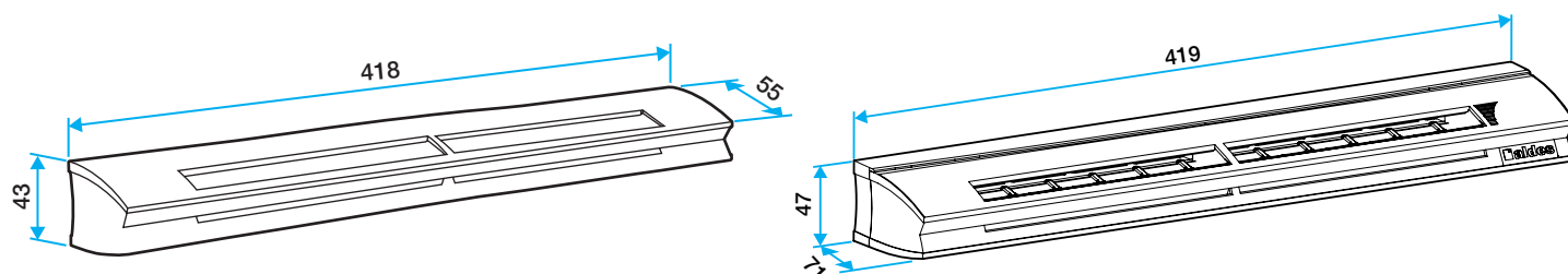
Montaje entrada de aire EHL S
