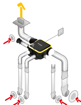
Instalación kit BIP con conductos rígidos Miniconducto
