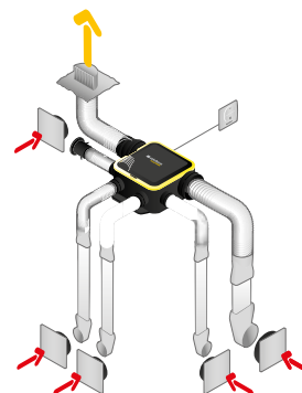
Instalación kit ColorLINE con conductos rígidos Miniconducto
