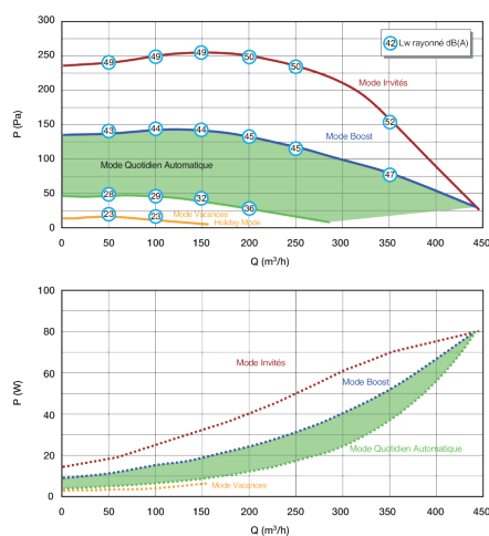
Curva aeráulica y acústica EasyHOME PureAIR COMPACT Premium
