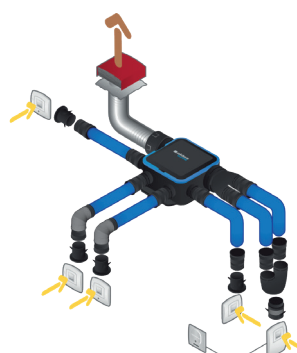
Instalación Easyhome Hygro Compact MW con bocas Bahia Curve y conducto Optiflex
