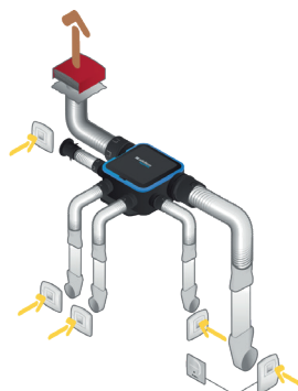
Instalación Easyhome Hygro Compact MW con bocas Bahia Curve y conducto Optiflex
