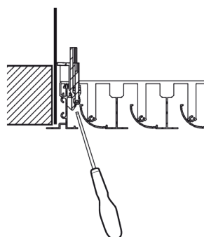
Difuseur de soufflage avec fixation S3
