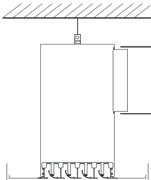
Difuseur de soufflage avec fixation S2
