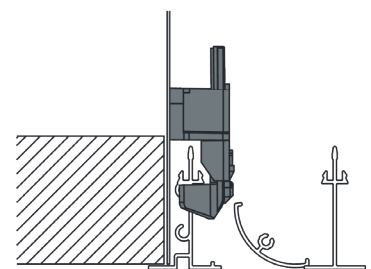
Gros plan fixation S3
