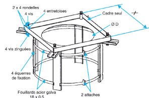
Marco en conducto VELONE
