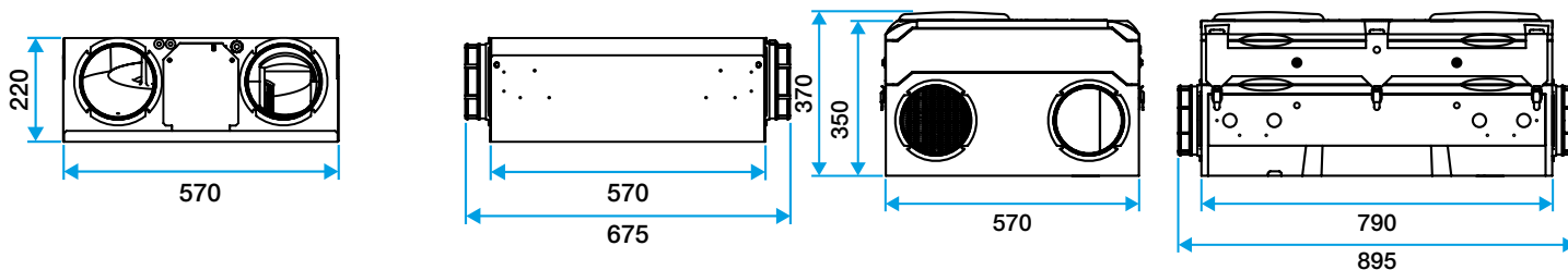
Moto-ventilateur
