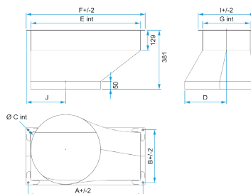
Pièce de transformation rectangulaire > circulaire VEX600
