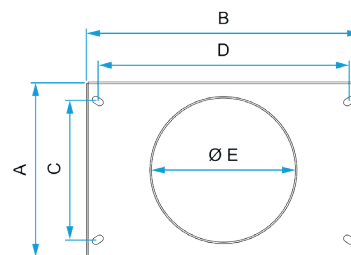
Pièce de transformation rectangulaire > circulaire VEX400
