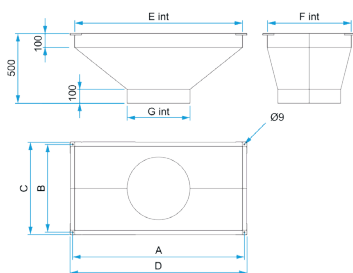
Pièce de transformation rectangulaire > circulaire VEX500
