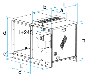
Encombremet ProtectONE® R EL 2V (mm)
