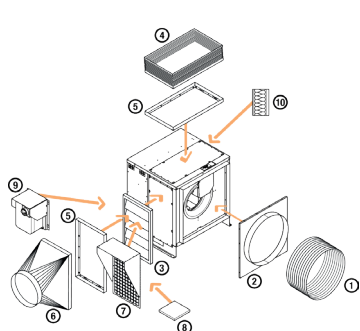
Options et accessoires ProtectONE® R (Modèle 90°)
