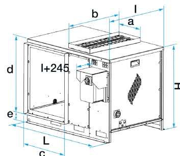
Encombrement ProtectONE® R EL 2V (mm)
