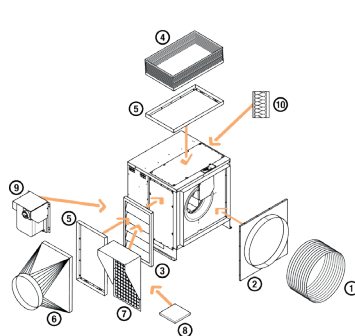
Options et accessoires ProtectONE® R (Modèle 90°)
