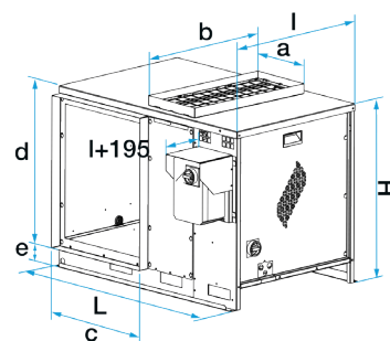
Encombremet ProtectONE® R EL 1V (mm)
