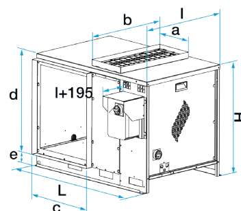
Encombrement ProtectONE® R EL 1V (mm)
