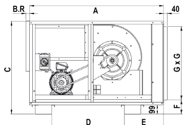
Encombremet (mm) - vue de profil
