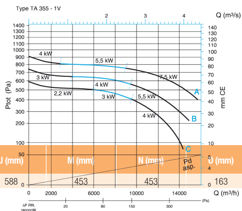
Características aeráulicas ProtectONE® TA 355 - 1V
