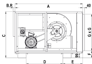
Dimensiones (mm) - vista de perfil
