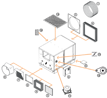
Accesorios ProtectONE T
