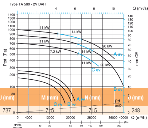
Características aerodinámicas del ProtectONE® TA 560 - 2V - DAH
