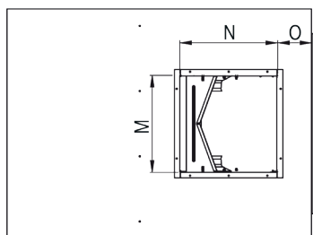
Dimensiones (mm) - vista superior
