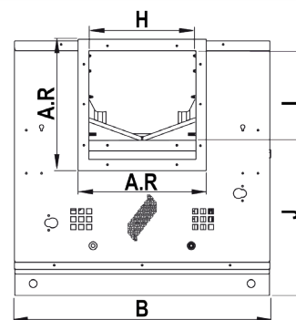
Dimensiones (mm) - vista frontal
