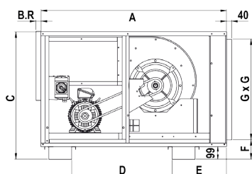
Encombremment (mm) - vue de profil
