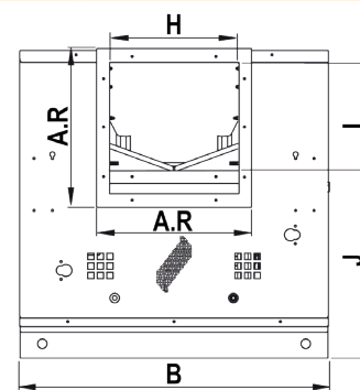
Encombremment (mm) - vue de face
