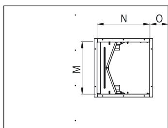
Encombremment (mm) - vue de dessus
