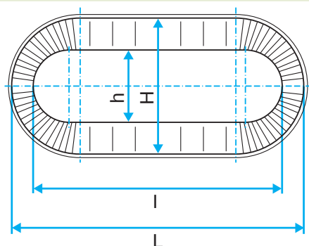
Esquema dimensiones Reducción Concéntrica Oblonga
