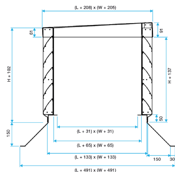
Remate AP 639 para cubierta plana (RF 639)
