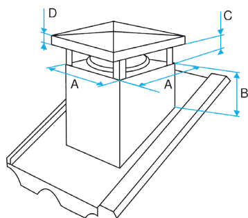
Schéma d'encombrement Sortie de Toit Esthétique
