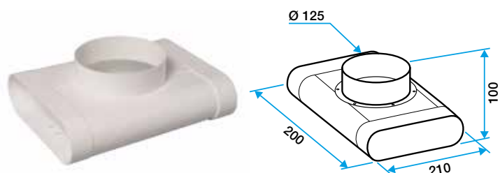
Té 90° vertical para boca
