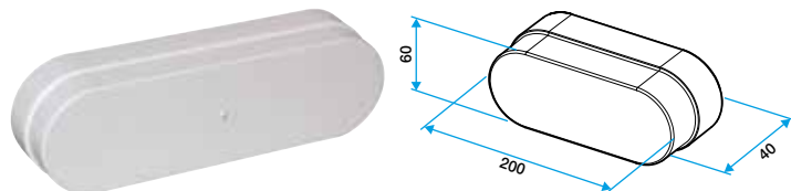
Tapa Miniconducto Ø125 mm
