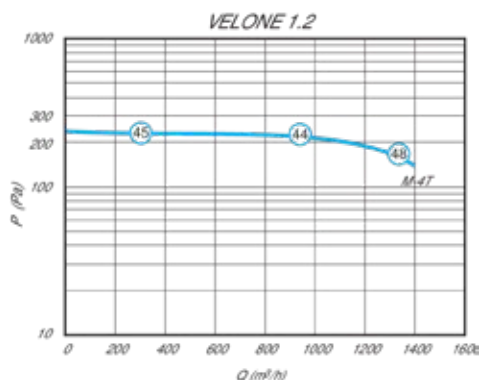
Caractéristiques aérauliques et acoustiques VELONE 1.2 - 4T 0.37 KW
