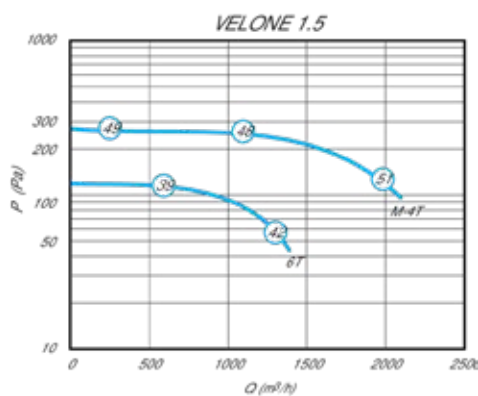
Caractéristiques aérauliques et acoustiques VELONE 1.5 - 4T 0.37 KW
