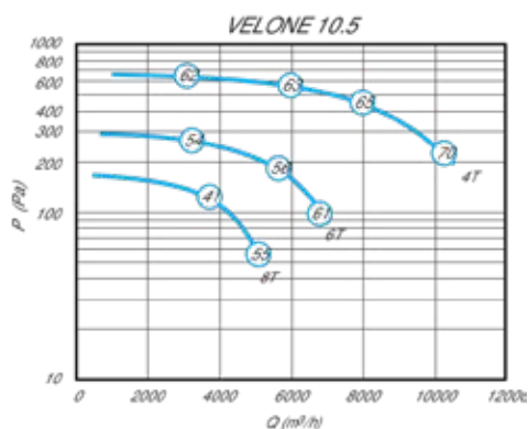
Características aerúlicas y acústicas de la VELONE 10.5 - 4T 1,5 KW
