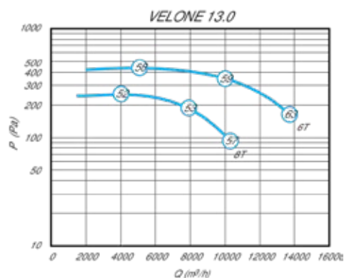
Características aeráulicas y acústicas de la VELONE 13 - 6T 2,2 KW
