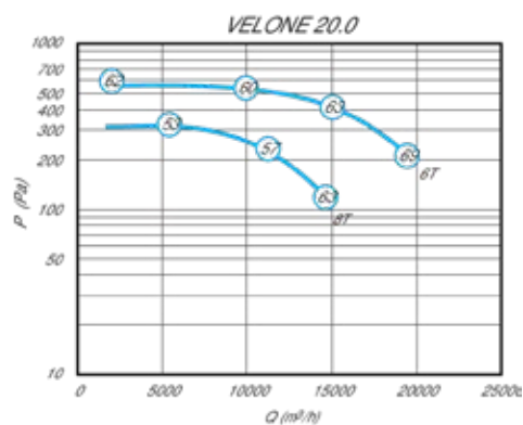
Características aeráulicas y acústicas de la VELONE 20 - 6T 3 KW
