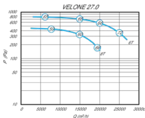
Características aerúlicas y acústicas de la VELONE 27 - 6T 5,5 KW
