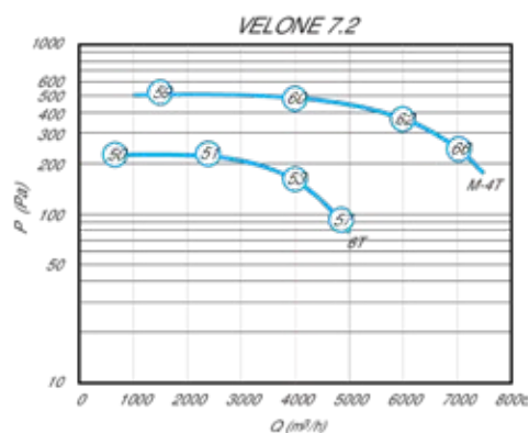
Características aeráulicas y acústicas de la VELONE 7.2 - 4T 1,1 KW
