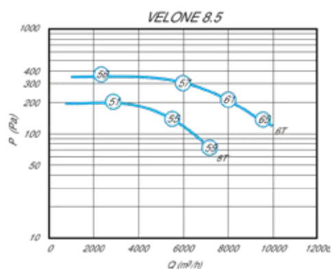
Características aerúlicas y acústicas de la VELONE 8.5 - 6T 1,1 KW
