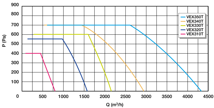
Características aerúlicas VEX300T
